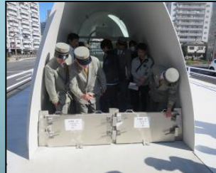
防潮板設置
